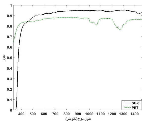
شکل ۴: تلف عبوری SU-8 (خط ممتد) و PET (نقطه چین) به صورت تابعی از طول موج
