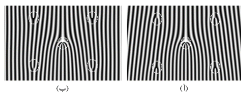
شکل ۱: توری چنگالی که فاصله‌ی تکینگی‌های فاز در آن برابر با d = \frac{\Lambda}{2} است. (ا) l_1 = +4, l_2 = +1 ، (ب) l_1 = +4, l_2 = -1
