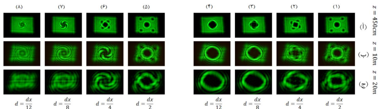
شکل ۳: نتایج تجربی، نمایه شدت برای تکینگی‌های فاز برابر با بارهای توپولوژیکی: تصویر سمت راست (۱-۴): l_1 = +4, l_2 = +1 و تصویر سمت چپ (۵-۸): l_1 = +4, l_2 = -1 . بازه‌ی نوار رنگ از ۰ تا ۲ و ابعاد پنجره نیز (5 \times 5 \text{ mm}) در نظر گرفته شده‌است.
