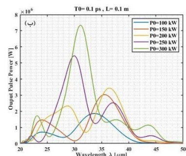
شکل ۴: طیف شبیه سازی شده (الف) پالس ورودی، (ب) ابرپیوستارخروجی
