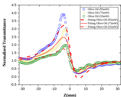
شکل ۴: نمودار تراگسیلندگی روزنه بسته نمونه زیتون
