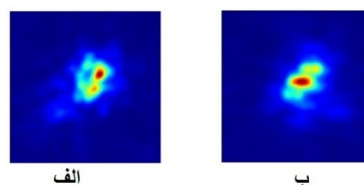
شکل ۸: (الف) توزیع شدت نور عبوری از جو، (الف) ناشی از یک ستاره در کانون تلسکوپ، (ب) ناشی از دو ستاره در کانون تلسکوپ.
