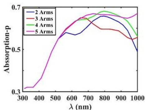
شکل (۲): طیف جذبی لایه نازک با طول ۳۰ و ۶۰ نانومتر، تعداد بازوی ۲ تا ۵ و زاویه تابشی و سمتی صفر درجه
