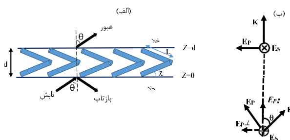
شکل (۱): (الف) نانوساختار زیگزآگی آلومینوم (ب) جهت گیری نور تابشی و مولفه های میدان الکتریکی
