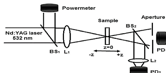
شکل ۳: طرح شماتیک از چیدمان آزمایشگاهی جاروب-Z
