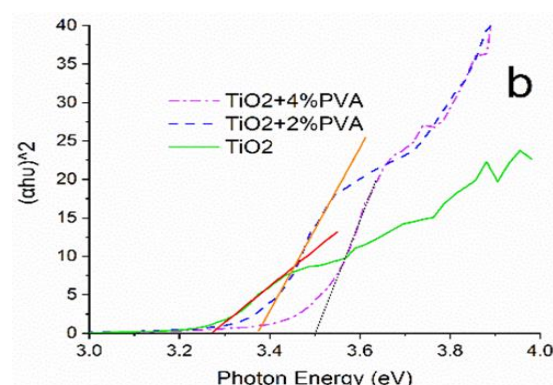
شکل 3-b: شکاف انرژی محاسبه شده برای نانو ذرات \text{TiO}_2 خالص و ترکیب شده با ۲ و ۴ درصد وزنی به روش تاک
