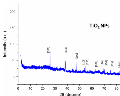
شکل ۱: الگوی پراش پرتو X نانو ذرات \text{TiO}_2
