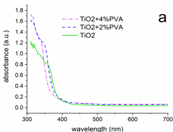
شکل 3-a: طیف سنج مرئی نانو ذرات \text{TiO}_2 خالص و ترکیب شده با ۲ و ۴ درصد وزنی
