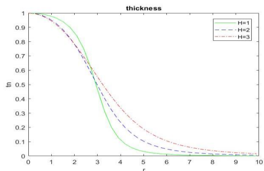
شکل ۳: محاسبه ضخامت لایه نشانی وابسته به شعاع برای D=4
