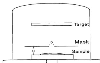
شکل ۲: طرح واره اجرای لایه‌نشانی متغیر
