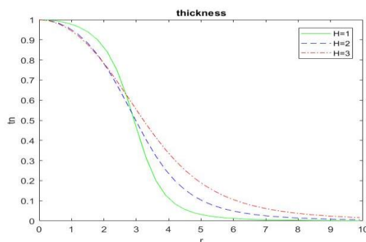
شکل ۳: محاسبه ضخامت لایه نشانی وابسته به شعاع برای D=۴
