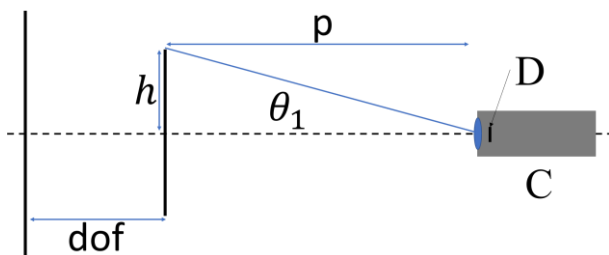
شکل ۱: هندسه قرارگیری دوربین. دوربین با نماد C، آشکارساز دوربین با نماد D، فاصله قرارگیری اولین دیواره از جسم با p و عمق میدان دید با dof، h نیم ارتفاع جسم، \theta_1 نیم زاویه میدان دید، معرفی شده است.
