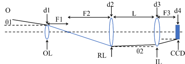
شکل ۲: چیدمان سیستم اپتیک. در این چیدمان، F1 فاصله کانونی عدسی شیئی، F2 فاصله کانونی عدسی میدان‌بند، F3 فاصله کانونی عدسی تصویر ساز، d1 قطر دهانه عدسی شیئی، d2 قطر دهانه عدسی میدان‌بند، d3 قطر دهانه عدسی تصویر ساز، D پهنای حسگر سی‌سی‌دی، L فاصله عدسی شیئی تا عدسی تصویر ساز، theta1 زاویه پرتو کناری رسیده به عدسی شیئی، theta2 زاویه خروج نور از عدسی میدان‌بند است.
