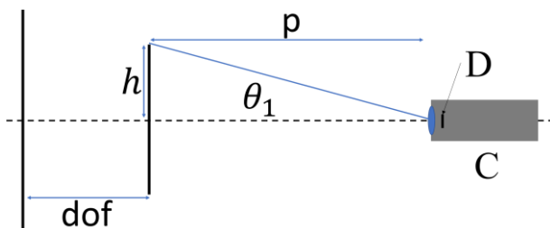
شکل ۱: هندسه قرارگیری دوربین. دوربین با نماد C، آشکارساز دوربین با نماد D، فاصله قرارگیری اولین دیواره از جسم با p و عمق میدان دید با dof، h نیم ارتفاع جسم، \theta_1 نیم زاویه میدان دید، معرفی شده است.
