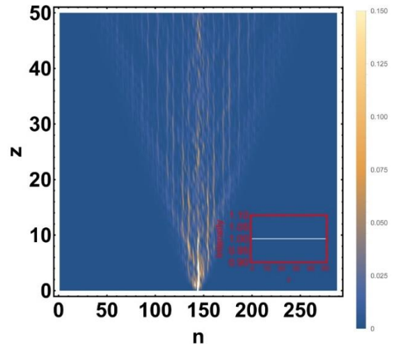
شکل ۲: الگوی انتشار نور برای \gamma = 0 یعنی وقتی که سیستم در فاز تقارن پاریته-زمان است. نمودار داخل شکل نحوه تغییر شدت بر حسب Z است که نشان می‌دهد شدت کل در طول انتشار ثابت می‌ماند.
