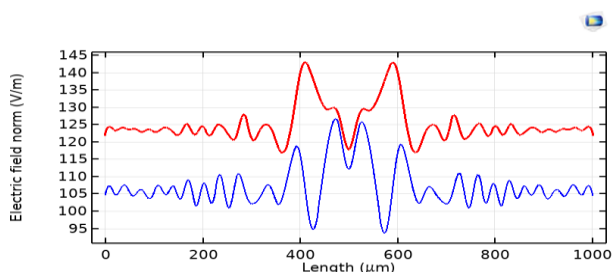
شکل 4: نمودار cut line برای طول موج 40 μm - نمودار قرمز رنگ عدم حضور سلول های توموری و نمودار آبی رنگ برای حالت توموری کردن سلول ها می باشد.
