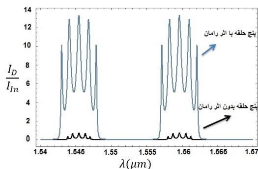
شکل ۵: مقایسه شدت انتقالی CROW پنج حلقه با وجود اثر رامان و بدون اثر رامان. کلیه ضرایب جفت‌شدگی ۰/۶ است.
