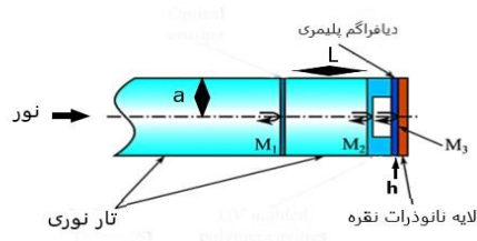
شکل ۱: شماتیک تداخل سنج فابری-پرو دیافراگمی
