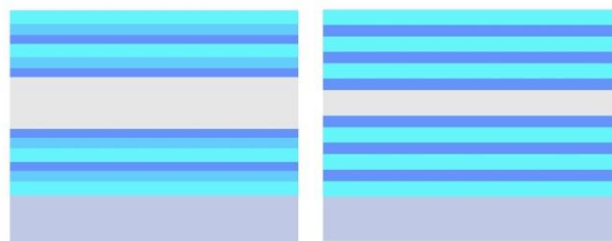
شکل ۲: بلور فوتونی یک-بعدي دو-ماده ای (راست) و سه-ماده ای (چپ) نقص دار با لایه های تخت
