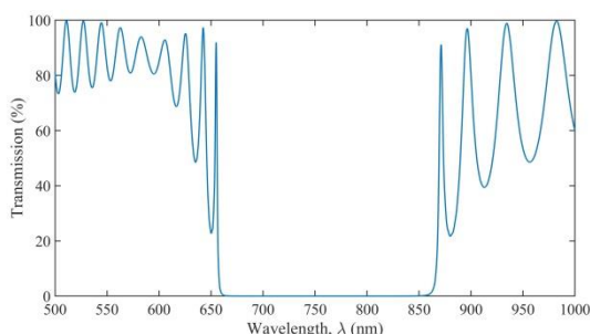
شکل ۴: طیف عبور بلور فوتونی یک-بعدي تخت دو-ماده ای بدون لایه نقص
