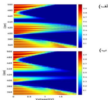
شکل ۳: طیف عبور امواج هم‌قطبش راستگرد به صورت تابعی از طول موج و ولتاژ الف) در حضور نانوذرات نقره، ب) در حضور نانوذرات طلا با f=0.00005 .
