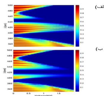
شکل ۳: طیف عبور امواج هم‌قطبش راستگرد به صورت تابعی از طول موج و ولتاژ الف) در حضور نانوذرات نقره، ب) در حضور نانوذرات طلا با f=0.0005 .
