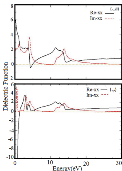
شکل ۴: بخش حقیقی و موهومی تابع دی‌الکتریک (الف) لایه خالص گرافن و (ب) لایه خالص گرافن با اتم ناخالصی بور.
