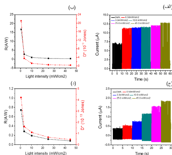
شکل ۳: نحوه تغییرات جریان بر حسب زمان تحت شدت های مختلف نور فرودی سفید رنگ با مقاومت 50\text{ M}\Omega برای آشکارساز خود مولد \text{SnS}_2/\text{PVK} بر پایه نانوذراتور الف) دست/FTO و ج) دست/FTO و تغییرات پارامترهای R^* و D آشکارساز نوری خودمولد بر حسب شدت های مختلف اعمالی نور سفید ورودی.
