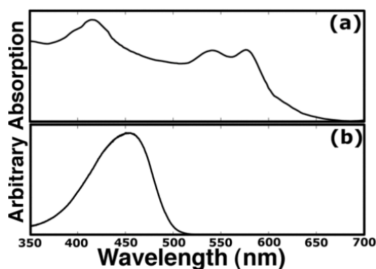
شکل ۳- طیف جذبی (a) هموگلوبین و (b) بیلی‌روبین
