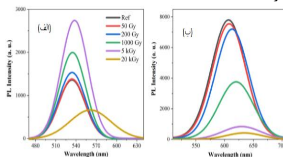
شکل ۴. الف) طیف نورتابی قبل و بعد از قرار گرفتن در معرض گاما برای (ب) CdTe و CdTe/CdSe/CdS
