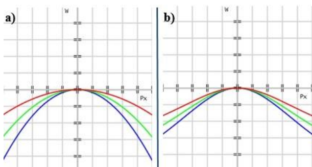
شکل ۶. اختلاف راه نوری را برای توری پراش نیم‌دایره (حداکثر مقیاس ۲ طول موج) (a) و توری پراش با خطوط خطی (b) را نشان می‌دهد.
