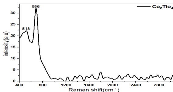
شکل (۲) طیف رامان نمونه \text{Co}_2\text{TiO}_3 .
