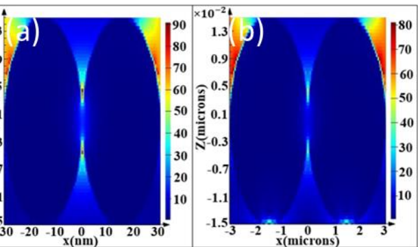
شکل ۲: (a) توزیع میدان الکتریکی در نانوذرات طلا بدون زیر لایه سیلیکون، (b) توزیع میدان الکتریکی در نانوذرات طلا با زیرلایه سیلیکون.
