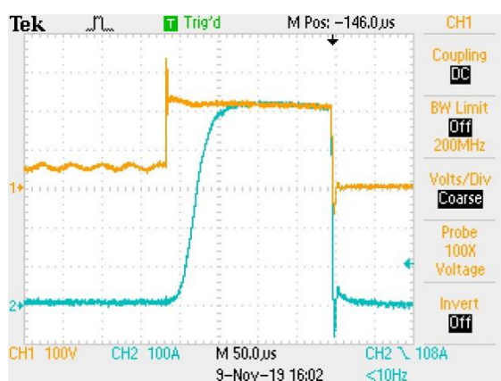
شکل ۳: ولتاژ (نسبت تضعیف ۲ به ۱) و جریان اندازه‌گیری شده برای فلاش لامپ ۸۵۳.
