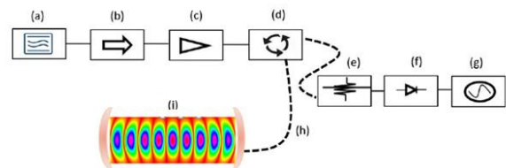
شکل ۲: نمای کلی الکترونیک میکروموج (a) ژنراتور سیگنال میکروموج، (b) یکسوساز، (c) تقویت کننده توان، (d) چرخاننده، (e) آنتن منطبق کننده، (f) آشکارساز دیود، (g) اسیلوسکوپ، (h) کابل SME کوکسیال، (i) شمایی از نوسانگر میکروموج با نقشه میدان الکتریکی مد در توان ۱۰ وات، [۴].
