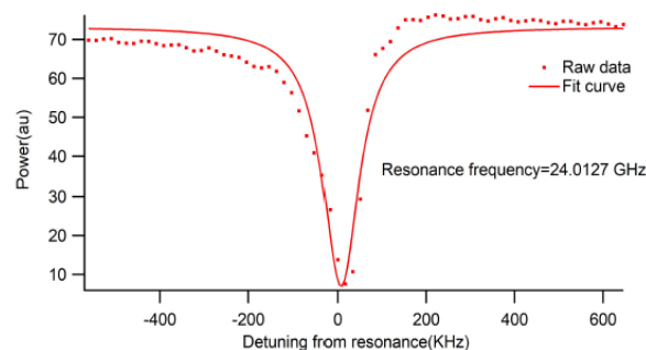
شکل ۳: طیف توان بازتابی اندازه گیری شده از کاواک MW.
