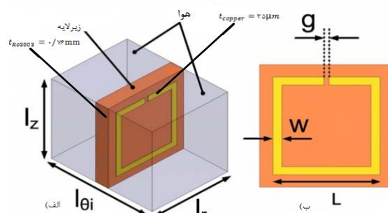
شکل ۳: طرحواره الف) سه بعدی. ب) دوبعدی سلول واحد پیشنهادی با مشخصات L_z = L_r = 4/5(mm) و L_{\theta} = 6(mm) و g = 0.18(mm) ، زیر لایه از جنس RO3003 با ضخامت t_{R03003} = 0.76mm و مشدد حلقوی شکافدار از جنس مس با ضخامت t_{copper} = 35\mu m می باشد.
