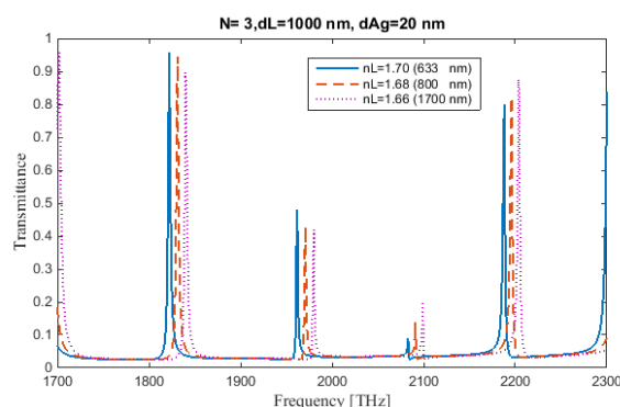
شکل ۵: مدهای نقص در سه طول موج ۶۳۳، ۸۰۰ و ۱۷۰۰ نانومتر برای ضریب شکست n_e
