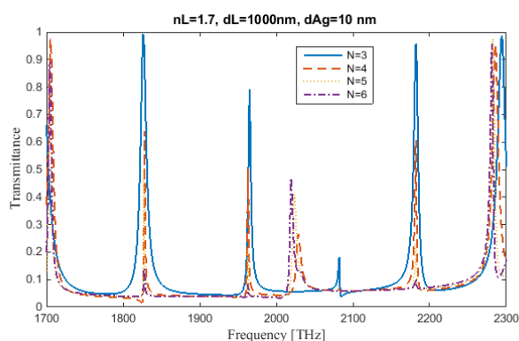
شکل ۲: مدهای نقص بلور فوتونی سه گانه بر حسب فرکانس
