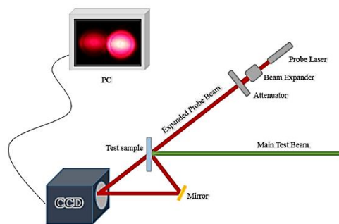
شکل ۲: شکل شماتیک از چیدمان تشخیص تخریب لیزری.
