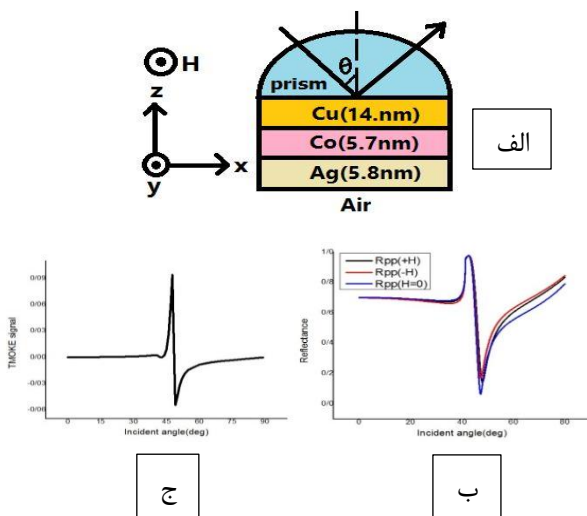
شکل ۱: قسمت الف شماتیکی از ساختار سه لایه معمول مگنتو-اپتیکی در پیکربندی کرشمن، قسمت‌های ب و ج به ترتیب منحنی‌های زاویه‌ای بدست آمده برای R(\pm H, H=0) و سیگنال TMOKE را نشان می‌دهند.
