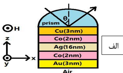
شکل ۱: قسمت الف شماتیکی از ساختار سه لایه معمول مگنتو-اپتیکی در پیکربندی کرشمن، قسمت‌های ب و ج به ترتیب منحنی‌های زاویه‌ای بدست آمده برای R(\pm H, H=0) و سیگنال TMOKE را نشان می‌دهند.
