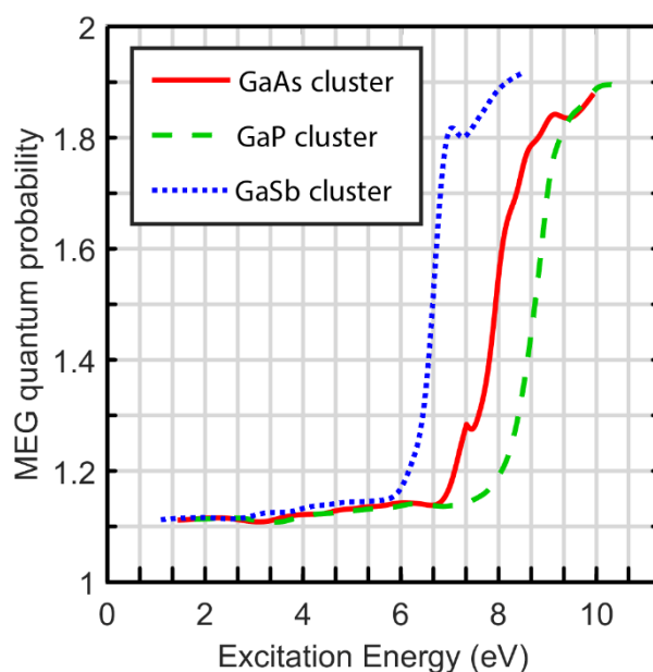
شکل ۲: نمودار احتمال کوانتومی MEG برای نانوخوشه های Ga 0.8 P 0.2 ، Ga 0.8 As 0.2 و Ga 0.8 Sb 0.2 برحسب الکترون - ولت
