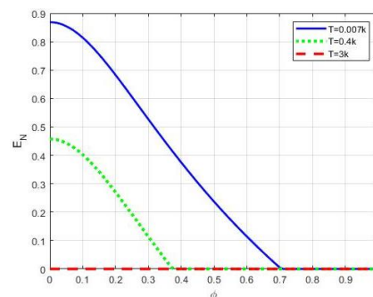
شکل ۵: درهم‌تنیدگی E_n بر حسب زاویه چلانیدگی \phi با دمای T مختلف زمانی که r=1 .
