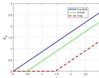
شکل ۴: درهم‌تنیدگی E_n بر حسب پارامتر چلانیدگی r با دمای T مختلف زمانی که \phi=0 .
