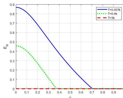
شکل ۵: درهم‌تنیدگی E_n بر حسب زاویه چلانیدگی \phi با دماهای T مختلف زمانی که r=1 .
