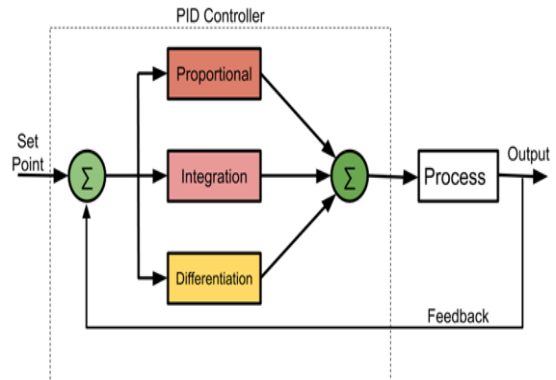
شکل ۲: طرحواره یک کنترل کننده PID
