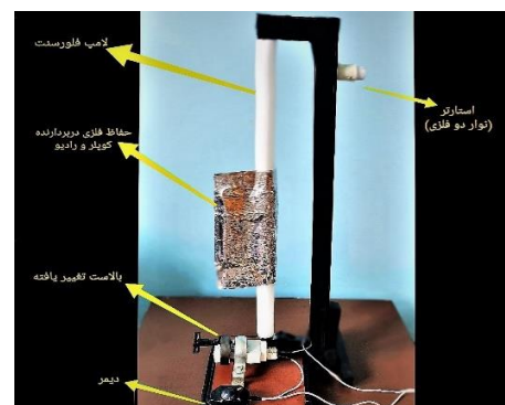
شکل ۴: نمای کلی از آنتن پلاسمایی ساخته شده
