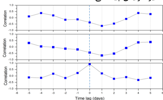
شکل ۵- نمودار ضرایب همبستگی برحسب تاخیرهای زمانی (۲۴ ژوئن ۲۰۱۰)، برای جفت سری های زمانی الف. AOD - دما ب. ARF - دما و ج. AOD - AR
