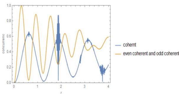
شکل ۲: درهم‌تنیدگی حالت خروجی اتمی بر حسب زمان برای حالت ورودی همدوس به ازای \omega = \omega_a = ۶۷۷۶۷ ، \omega = ۱ ، g = ۱۴۸۸۳۳ ، \theta = ۱ و \alpha = ۴۱۴۱ ، برای حالت ورودی همدوس زوج به ازای \omega = \omega_a = \theta = ۱ ، g = ۳۰۸۸۱۶ و \alpha = ۲۵۴۹۲ و حالت ورودی همدوس فرد به ازای \omega = \omega_a = \theta = ۱ ، g = ۳۰۸۸۰۲ و \alpha = ۲۵۵۶۸ .
