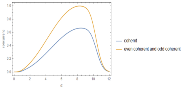
شکل ۱: درهم‌تنیدگی حالت خروجی اتمی بر حسب پارامتر همدوسی برای حالت ورودی همدوس به ازای \omega = \omega_a = ۶۷۷۶۷ ، \omega = ۱ ، g = ۱۴۸۸۳۳ ، \theta = ۱ و t = ۶۲۸۶۰۸ ، برای حالت ورودی همدوس زوج به ازای \omega = \omega_a = \theta = ۱ و g = t = ۳۰۸۸۱۶ و حالت ورودی همدوس فرد به ازای \omega = \omega_a = \theta = ۱ و g = t = ۳۰۸۸۰۲ .
