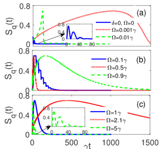
شکل ۴: آنتروپی کیوبیت (S_q(t)) به ازای زمان بی بعد \gamma t .
