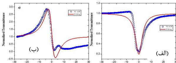
شکل ۲: نمودار تراگسیلندگی بهنجار عبوری جاروب محوری با برازش برای توان ۹۵ میلی‌وات کادمیم تلوراید آلائیده شده با منگنز با ساخت ۴ ساعت و برازش هر یک با استفاده از روابط (الف) (۵) و (ب) (۶)
