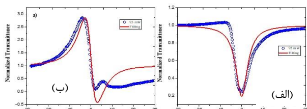
شکل ۲: نمودار تراگسیلندگی بهنجار عبوری جاروب محوری با برازش برای توان ۹۵ میلی‌وات کادمیم تلوراید آلائیده شده با منگنز با ساخت ۴ ساعت و برازش هر یک با استفاده از روابط (۵) و (۶)
