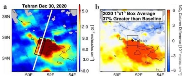
شکل ۵: (a) توزیع فضایی \text{NO}_2 استخراجی سنجنده OMI در روز ۳۰ دسامبر ۲۰۲۰ و گذر CALIPSO. (b) اختلاف توزیع فضایی \text{NO}_2 نسبت به میانگین \text{NO}_2 در مدت مشابه ۵ سال قبل (۲۰۱۵-۲۰۱۹).
