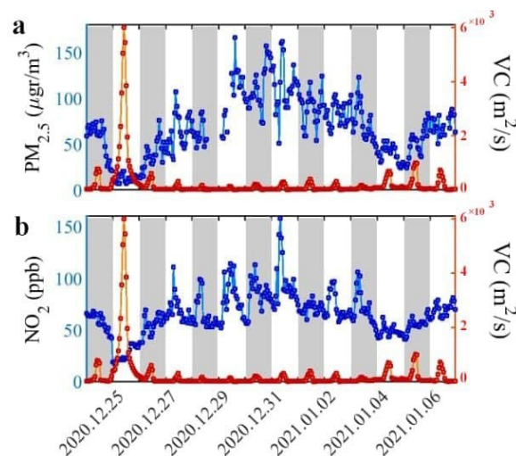
شکل ۶: نمودار ساعتی آلاینده‌های (a) \text{PM}_{2.5} و (b) \text{NO}_2 دریافتی از شرکت کنترل کیفیت هوای شهر تهران طی بازه ۲۴ دسامبر ۲۰۲۰ الی ۶ ژانویه ۲۰۲۱ میلادی.
