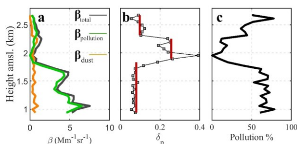
شکل ۶: نمایه قائم (a) ضریب پس‌پراکنش 532\text{nm} ، (b) ضریب واقطبش و (c) درصد آلودگی در گذر عبوری CALIPSO روز ۳۰ دسامبر ۲۰۲۰ بر فراز استان تهران.
