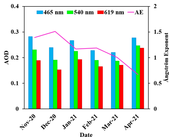
شکل ۳: تغییرات میانگین ماهانه AOD در ۳ طول موج ۴۶۵، ۵۴۰، ۶۱۹ نانومتر و میانگین ماهانه AE در طول موج ۴۶۵-۶۱۹ نانومتر.
