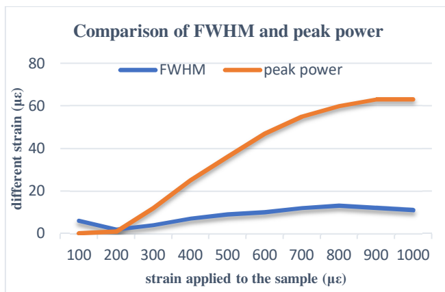
شکل ۲- نمودار فیت‌شده دو روش FWHM و توان پیک بازتابی با توجه به جدول ۱
