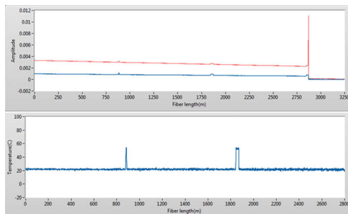
شکل ۲: بخشی از پانل کاربری حسگر ساخته شده، بالا- سیگنال‌های دریافتی استوکس (قرمز) و پاداستوکس (آبی) از فیبری به طول ۳ کیلومتر که دو پیچیه به طول‌های ۷ و ۱۸ متر در فواصل ۸۸۰ متر و ۱۸۶۰ متری در دمای ۵۵ درجه سانتی‌گراد قرار گرفته است. و ب- پروفایل دمایی این فیبر.
