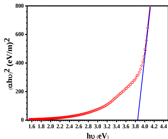
شکل ۶: نمودار (\alpha h\nu)^2 بر حسب انرژی فوتون برای لایه نازک تیتانیوم دی‌اکسید تهیه شده با روش چرخشی
