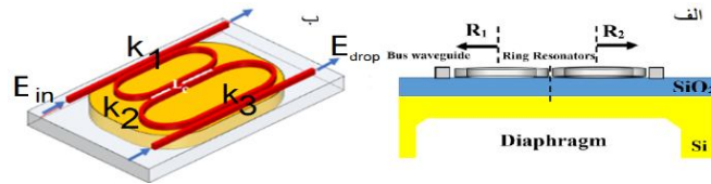
شکل ۱: نمای کلی از حسگر فشار بر پایه تشدیدگر حلقوی (الف) پیکر بندی موجبری (ب) نمای حلقه سیلیکونی روی دیافراگم مستطیلی
